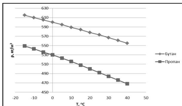
Рис. 1. Залежність густини бутану і пропану від температури
