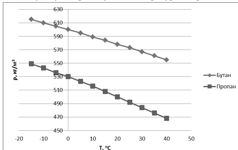
Рис. 1. Залежність густини бутану і пропану д температури
