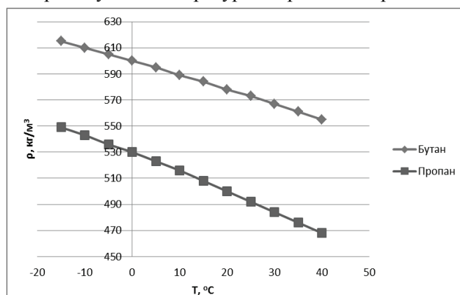
Рис. 1. Залежність густини бутану і пропану від температури
