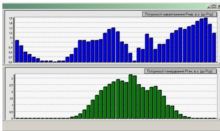
Рис. 1 – Типові графіки навантаження та генерування у відносних одиницях (за базис прийнято середнє навантаження/генерування)
