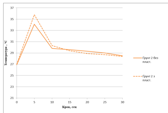
Рис. 4. Температурні криві охолодження досліджуваного ґрунту № 2
