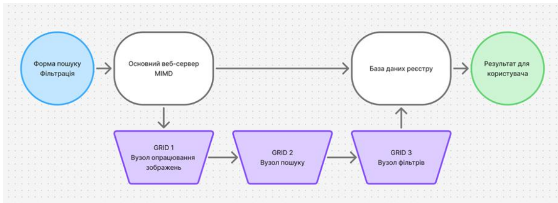
Рисунок 1 – Нова структура опрацювання даних
