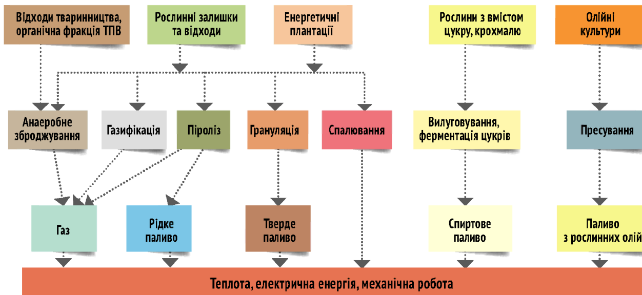
Рис. 2. Способи виробництва енергії з біомаси
