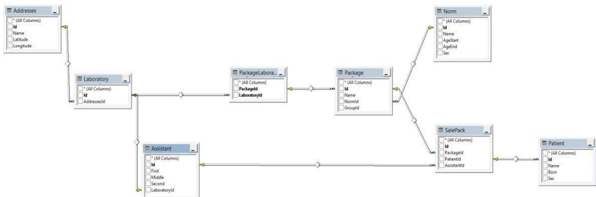
Рисунок 2 – Структурна схема бази даних консолідованого ресурсу
