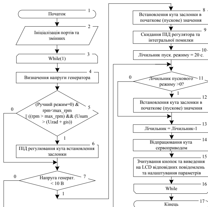
Рис. 1. Алгоритм функціонування мікропроцесорного блоку керування мобільною енергетичною установкою
