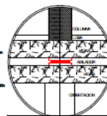
Схема ізоляційної системи
