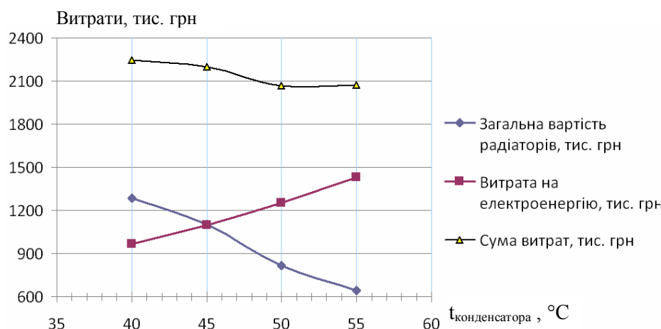
Рисунок 1 – Залежність витрат при роботі теплового насоса «вода-вода» з радіаторною системою опалення від температури теплоносія на виході з конденсатора
