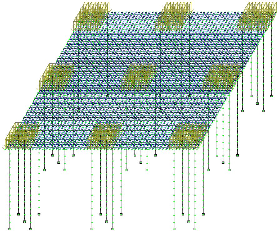
Рис. 2. Загальний вигляд розрахункової моделі у варіанті моделювання куців паль, об'єднаних суцільною фундаментом плитою
