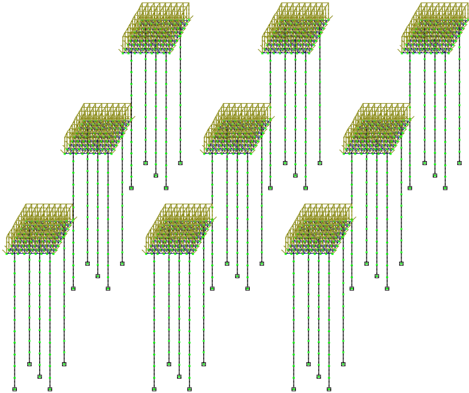
Рис 1. Загальний вигляд розрахункової моделі у варіанті моделювання тільки куців палей, що сприймають навантаження
