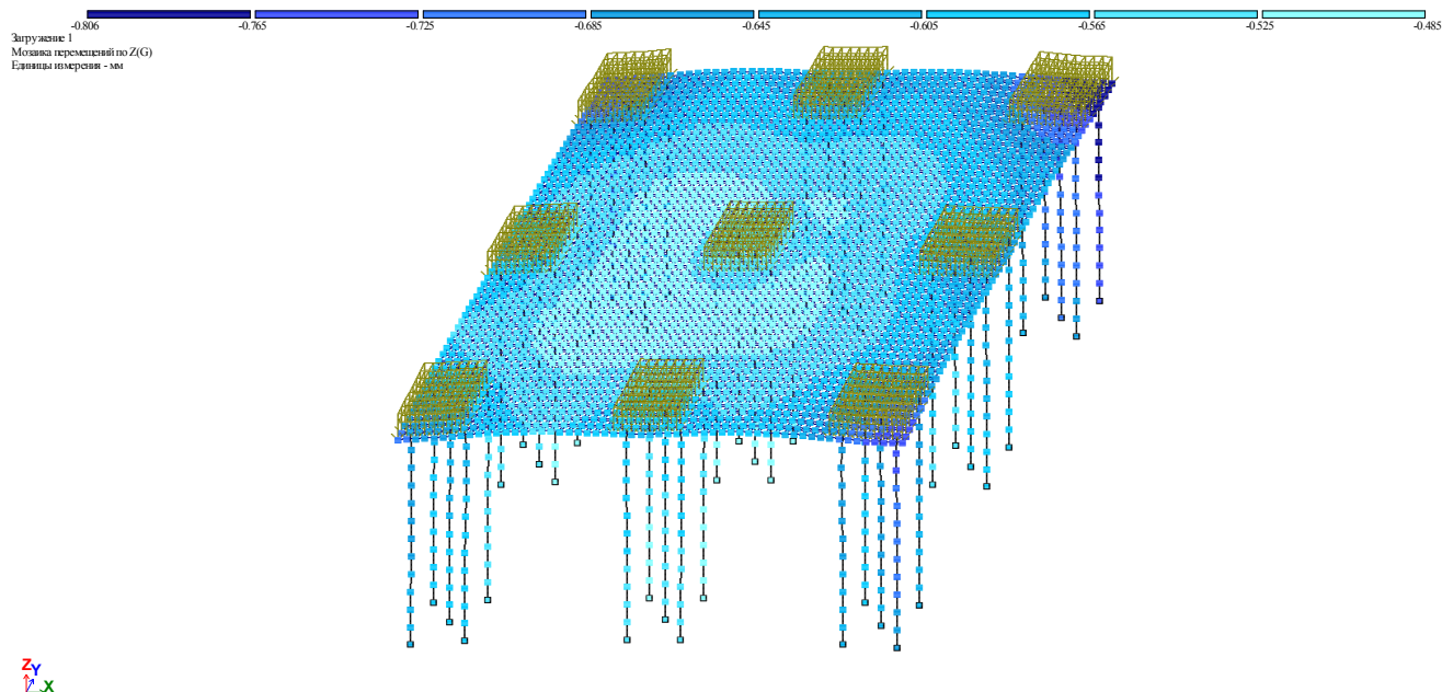
Рис. 4. Деформована схема розрахункової моделі у варіанті моделювання куців паль, об'єднаних суцільною фундаментною плитою
