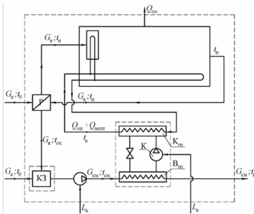
Рис. 1. Принципова теплонасосно-рекуператорна схема опалення та вентиляції з використанням теплоти вентиляційного і атмосферного повітря: К тн – конденсатор ТН; В тн – випарник ТН; К – компресор; В – вентилятор; КЗ – камера змішування; Р – рекуператор.
