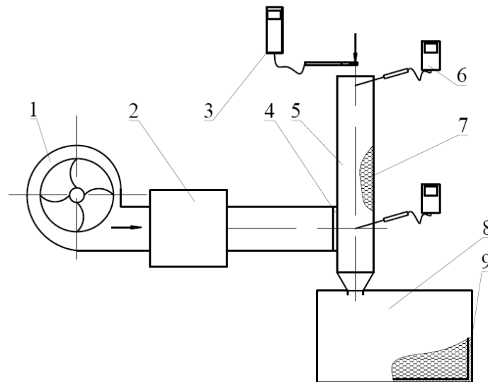
Рис. 1. Установа для експериментального дослідження теплообміну в щільному шарі гранульованого матеріалу: 1 – вентилятор; 2 – нагрівник; 3 – анемометр; 4 – сітка; 5 – робоча камера; 6 – термометр; 7 – гранульований матеріал; 8 – ємність збору дисперсного матеріалу; 9 – ізоляція
