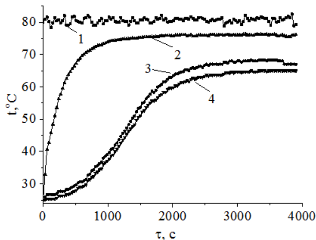
Рис. 3. Зміна температури повітря і керамзиту у часі: 1 – температура повітря на вході в апарат; 2 – температура матеріалу за x = 0 м; 3 – температура повітря на виході з апарату; 4 – температура матеріалу за x = 0,52 м; w_{ф} = 1,0-2,0 м/с; t'_{п} = 80 °C; L = 0,52 м; m = 5,25 кг
