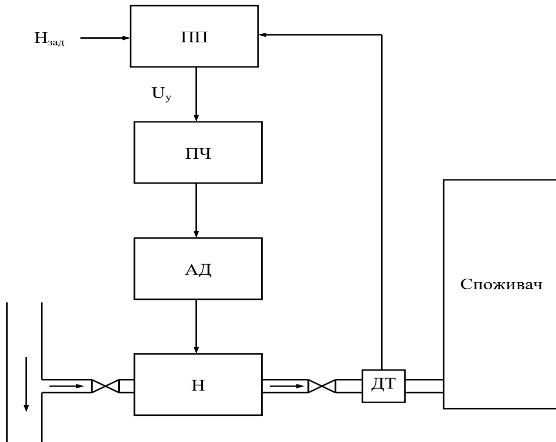
Рисунок 2 - Функцїональна схема системи автоматичного керуваннн ПЧ-АД
