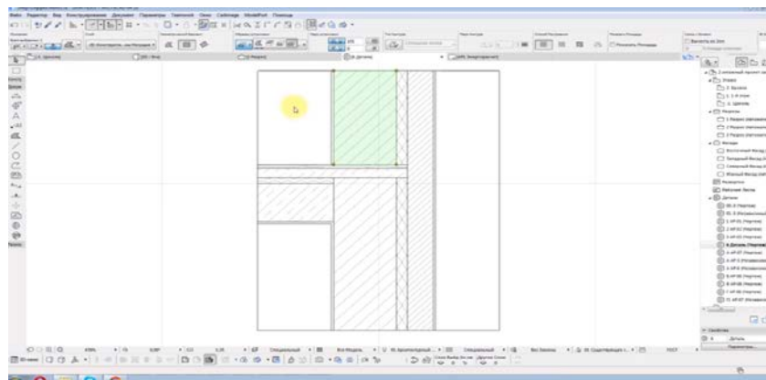
Рис. 2. – Вузол обпирання плити перекриття на цегляну стіну.
