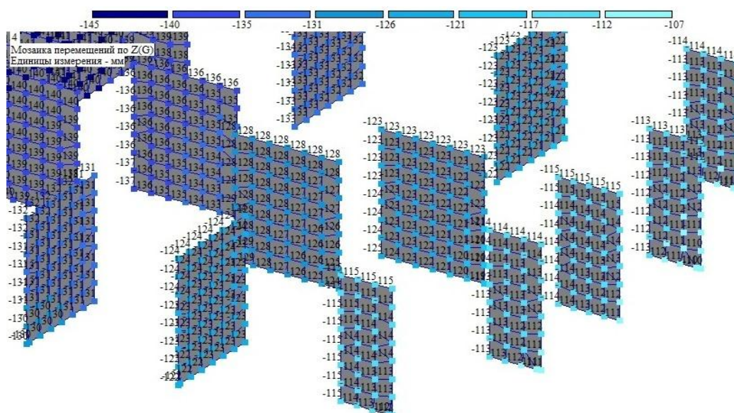
Рис. 1 - Деформований стан
