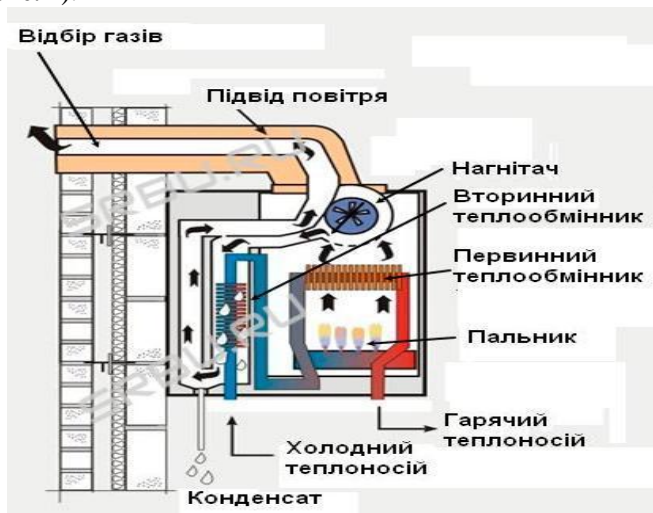
Рис. 2. Принципова схема роботи конденсаційного котла
