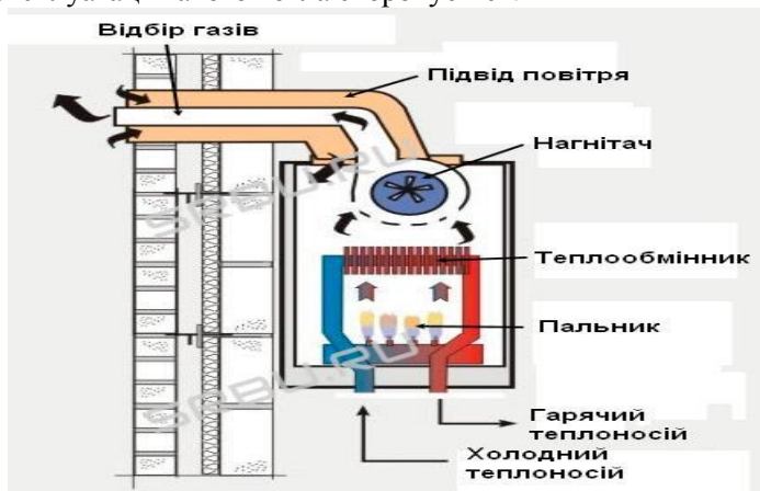
Рис. 1. Фрагмент конвекційного котла змонтованого на стіні
